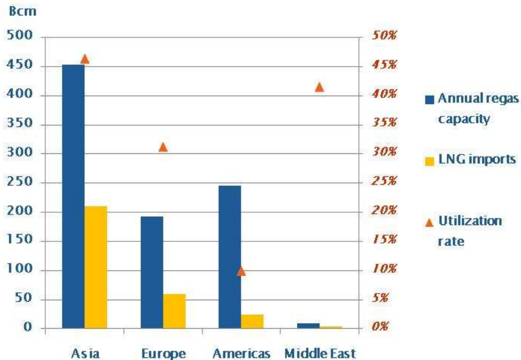
Regasification capacity vs LNG imports in 2012
